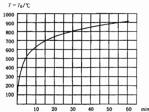
图 A.3 时间-温度标准曲线
